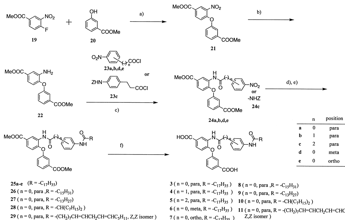
Scheme 1. Condition: (a) K 2 CO 3 /DMF, 92%; (b) H 2 /Pd-C; (c) 23a–e , Et 3 N, 19–100% from 21 ; (d) H 2 /Pd-C; (e) RCOCl, Et 3 N, 8–79% from 24a–e ; (f) 1 N NaOH, 9–99%.
